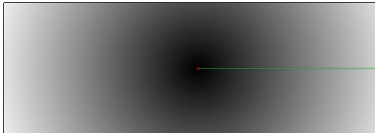
Radial Gradient
