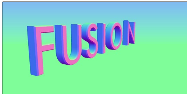
XYZ Normals
