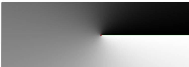
Angle Gradient
