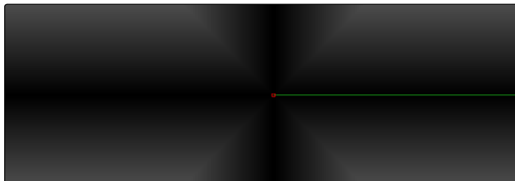
Cross Gradient
