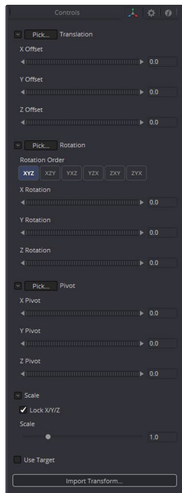
Transformation tab
